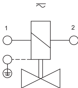
Anschlußplan/ Wiring diagram
