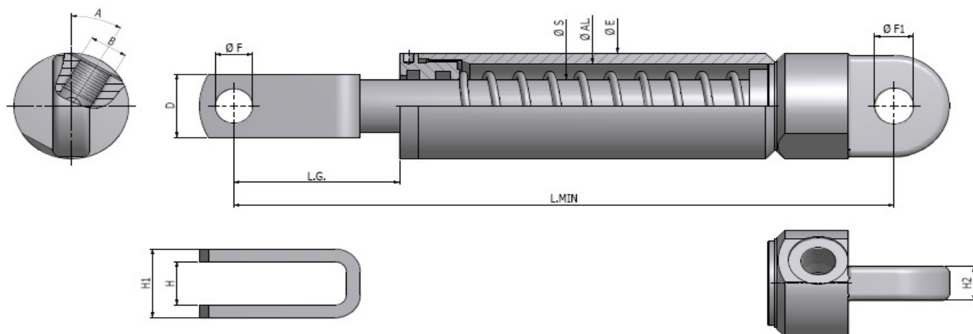
CILINDRO TIPO BRAKE CYLINDER
