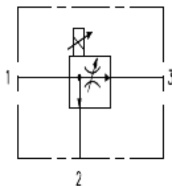
HG755-3 CAV TVTP90
