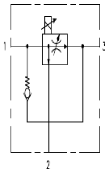
HG755-1 CAV TVTP90
