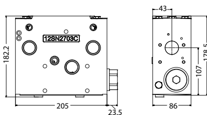
PVB 256 basic module dimensions (mm)
