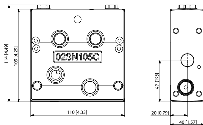
PVB 16 dimensions
