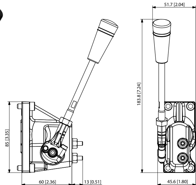
PVM dimensions
