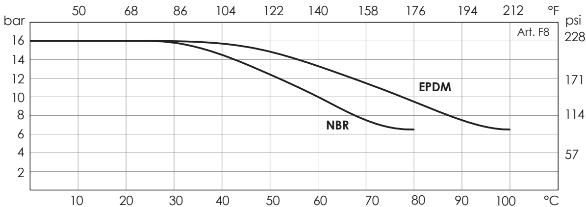
Druck-Temperatur Diagram Gewinde/ Pressure-Temperature Diagram thread
